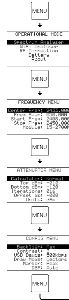
Schéma 4 Structure du menu
