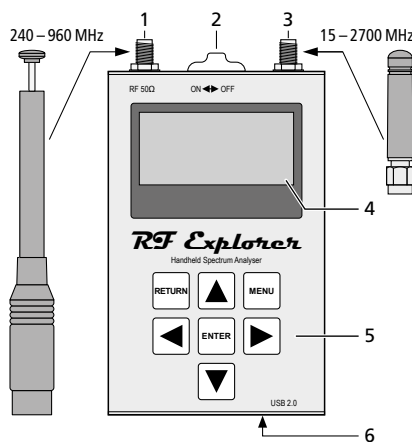
Fig. 1 Collegamento e elementi di comando
