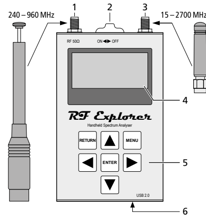
Abb. 1 Anschlüsse und Bedienelemente
