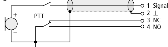
① DH-95N
