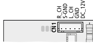
Leiterplatte mit Anschlüssen
